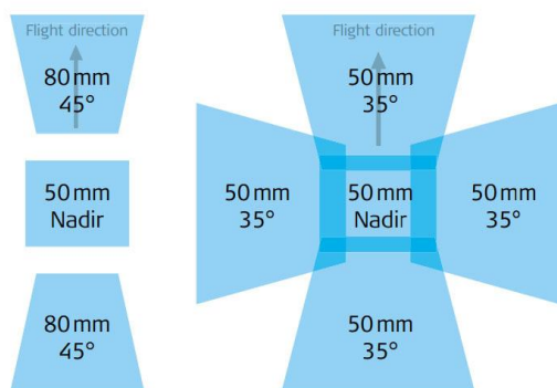
Схема съемки камерами RCD30 Oblique Trio и RCD30 Oblique Penta
